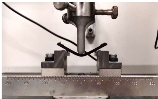
Preverjanje mehanskih lastnosti BioTHOP kompozita
