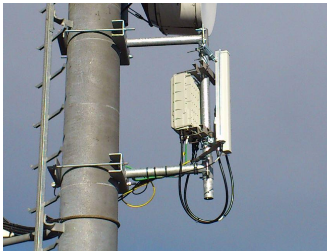
namestitev anten na postaji OŠO
