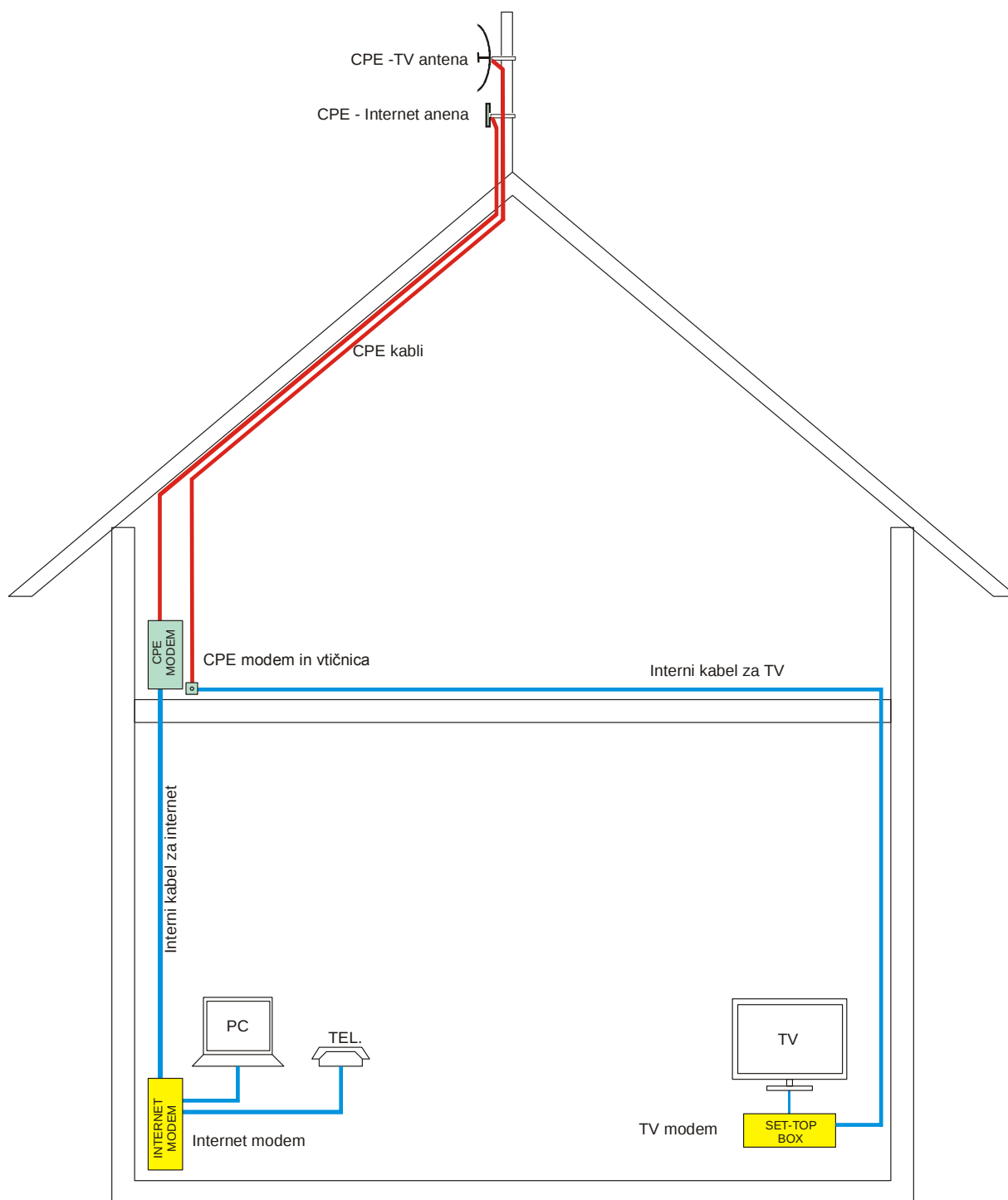
tipičen primer namestitve opreme v/na objektu
